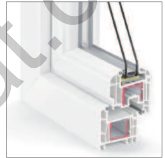
Oval Kanat Dizaynı
