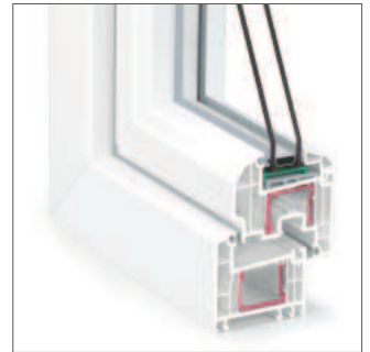
A Kanat Dizaynı
